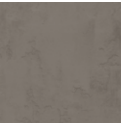
Fog
